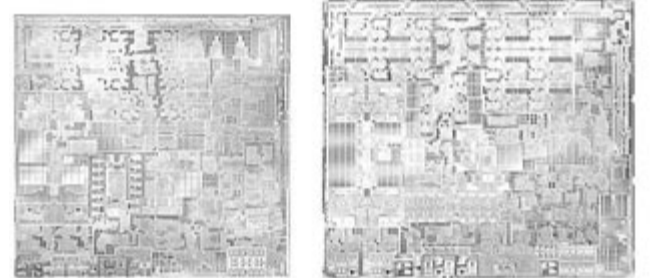
Az Apple M1 és M2 processzorainak felépítése
