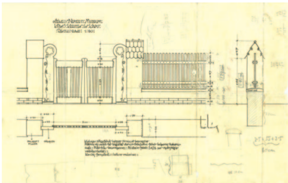
A külső kerítés és kapu részletrajza, 1912
