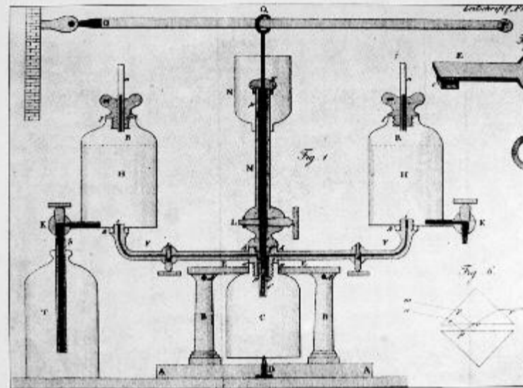
Jedlik szódavíz készítő gépe. Rékeslet a Zeitschrift für Physik und Mathematik 1830-as 7. évfolyamán 1. képfelirásból. melében a fig. 1. ábratáján Jedlik gépét.
