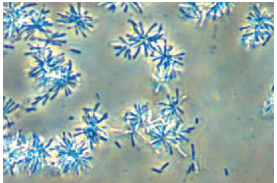
A Siculibacillus lacustris SA-279 kódjelű típus törzsének rozettákat formáló sejtjei fénymikroszkópos fáziskontaszt felvételen, százsoros nagyításban. A sejtek hossza 1,3-2,5 µm.
