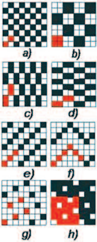
Különböző egyszerű szövet-kötésmódok. a) – vászonszőtés, b) – panamakötés, c) – láncrisz, d) – vetülékrisz, e) sávolykötés, f) – ék alakú sávoly, g) – láncatlasz, h) – vetülékatlan
